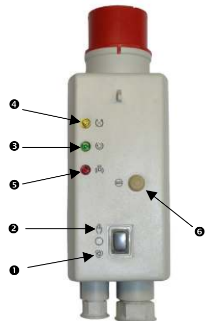
Bild 3: Schwimmerschalter-Motorschutzstecker
